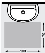
Умывальник
