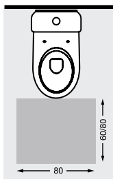
Унитаз
