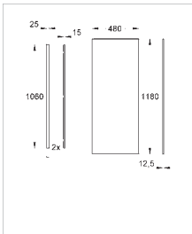
38 630 001 Rapid SL облицовочная панель для биде, писсуара и свободного пространства между элементами, монтажная высота 1.13 м, без отверстий
