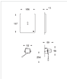
38 699 000 Tectron Surf для смывного бачка GD 2, скрытая установка, инфракрасное управление, 230 V, сервопривод, накладная панель: хром
