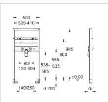
38 541 000 то же, что и 38 625 001, монтажная высота 1.00 м., без сифона
