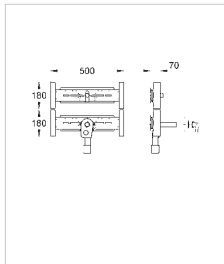
38 441 000 Rapid SL держатель смесителя для стиральной машины, для стен-перегородок из гипсокартона
