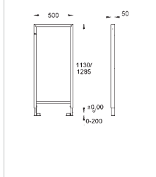
38 548 001 Rapid SL пустой элемент монтажная высота 1.13 м, для установки держателей арматуры
