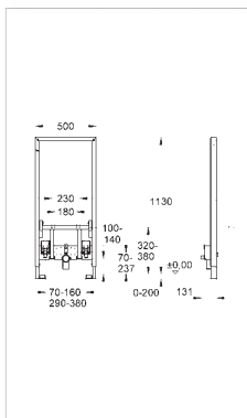
38 553 001 Rapid SL для биде монтажная высота 1.13 м
