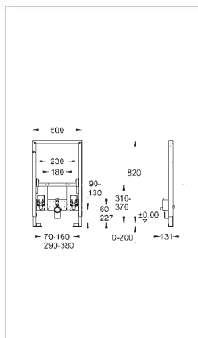
38 543 000 Rapid SL для биде монтажная высота 0.82 м
