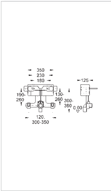
37 576 001 Uniset для биде
