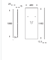
38 631 001 Rapid SL облицовочная панель для раковины, высота установки 1.13 м, с пазами
