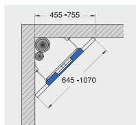
Rapid SL для умывальника, 1.13 м
