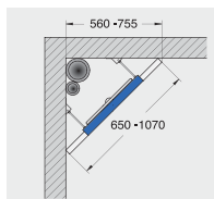
Rapid SL для писсуара со смывным устройством 37 338 000 (ручное управление), монтажная высота 1.13 м
