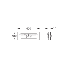
37 999 000 Rapid SL держатель смесителя для настенных смесителей, для стен-перегородок и пустых элементов
