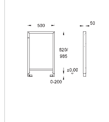
38 551 000 Rapid SL пустой элемент то же, что и 38 548 001, но монтажная высота 0.82 м/1.00 м
