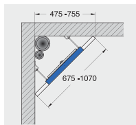
Rapid SL для писсуара Joly/ Visit, для писсуара Joly/Visit со смывным устройством 37 338 000 (механический смыв), монтажная высота 1.13 м
