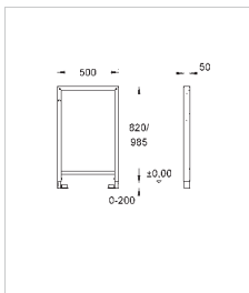
38 551 000 Rapid SL то же, что и 38 548 001, но монтажная высота 1.00 или 0.82 м
