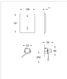
38 698 SD0 Tectron Skate для смывного бачка GD 2, скрытая установка, инфракрасное управление, 230 V, сервопривод, накладная панель: нержавеющая сталь
