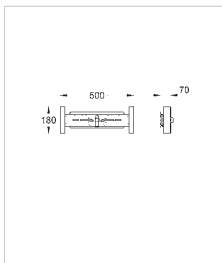
37 999 000 Rapid SL держатель смесителя для настенного монтажа, для стен-перегородок и пустых элементов
