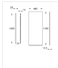
38 630 001 Rapid SL облицовочная панель для писсуара, биде и пространства между элементами, монтажная высота 1.13 м, без отверстий
