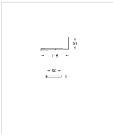
43 617 000 Кронштейн для двигателя Rapid SL 38 675 001, для установки инфракрасной электроники
