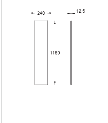
38 633 001 Rapid SL облицовочная панель для боковой стороны/выступов для монтажной высоты 1.13 м, 1.00 м и 0.82 м
