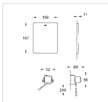
38 559 001 Элемент-держатель Rapid SL для опорных поручней на стенах-перегородках или монтажа перед стеной
