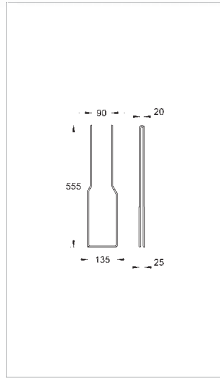
37 573 000 Uniset вертикальные кронштейны для унитаза и биде, для свободно стоящей установки (не подходят для монтажной высоты 0.82 м)
