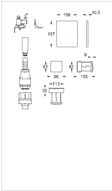
38 564 000 Накладная панель Skate Air 1 объем смыва, 156 x 197 мм, вертикальная установка, из ABS, для пневматического смывного клапана
