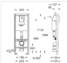
38 675 001 Rapid SL для подвесного унитаза со смывным бачком 6 л, два объема смыва, функция start/stop, монтажная высота 1.13 м, ширина 0.42 м,
