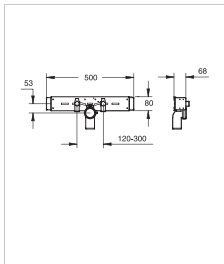
38 437 000 Rapid SL держатель смесителя для мойки, для стен-перегородок, 2 звукоизоляционных подключения смесителя
