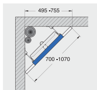
Rapid SL для унитаза, со смывным бачком GD 2, 1.13 м
