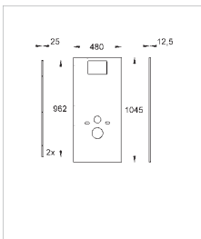
38 637 001 Rapid SL облицовочная панель монтажная высота 1.00 м
