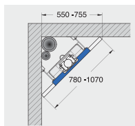
Rapid SL для унитаза, со смывным бачком 0.82 или 1.00 м
