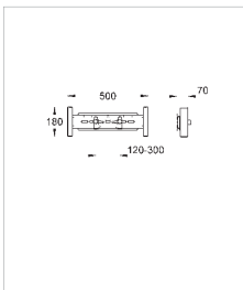
37 998 000 Rapid SL держатель смесителя для настенного монтажа, для стен-перегородок и пустых элементов
