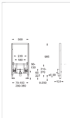
38 545 000 Rapid SL для биде монтажная высота 1.00 м
