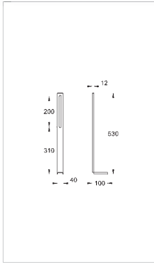
37 304 000 Uniset несущие стойки для унитаза и биде, для монтажа перед стеной
