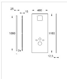
38 636 001 Rapid SL облицовочная панель для унитазов, монтажная высота 1.13 м
