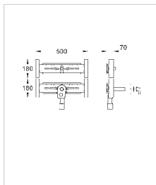
38 441 000 Rapid SL держатель смесителя для стиральной машины, для стен-перегородок и пустых элементов
