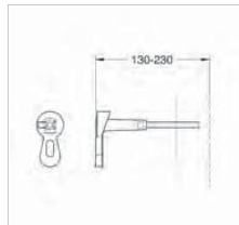
38 558 000 Rapid SL настенный уголок для монтажа перед стеной, 2 штуки
