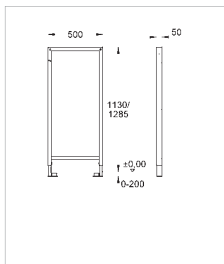
38 548 001 Rapid SL Пустой элемент Монтажная высота 1,13 м Для инсталляции с отдельностоящим элементом
