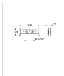
37 998 000 Rapid SL держатель смесителя для настенных смесителей, для стен-перегородок и пустых элементов
