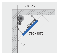
Rapid SL для писсуара Joly/ Visit, для писсуара Joly/Visit со смывным устройством 37 338 000 (механический смыв), монтажная высота 1.13 м
