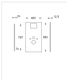
38 638 000 Rapid SL облицовочная панель монтажная высота 0.82 м
