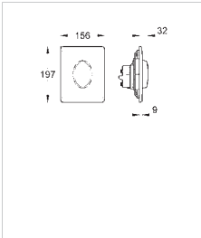
38 564 000 Накладная панель Skate Air 1 объем смыва, 156 x 197 мм, вертикальная установка, из ABS, для пневматического смывного клапана
