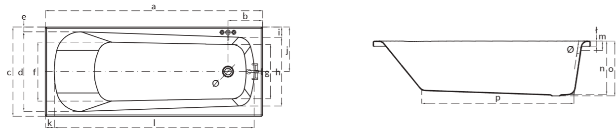
Прямокутна ванна NAO NAO rectangular bathtub
