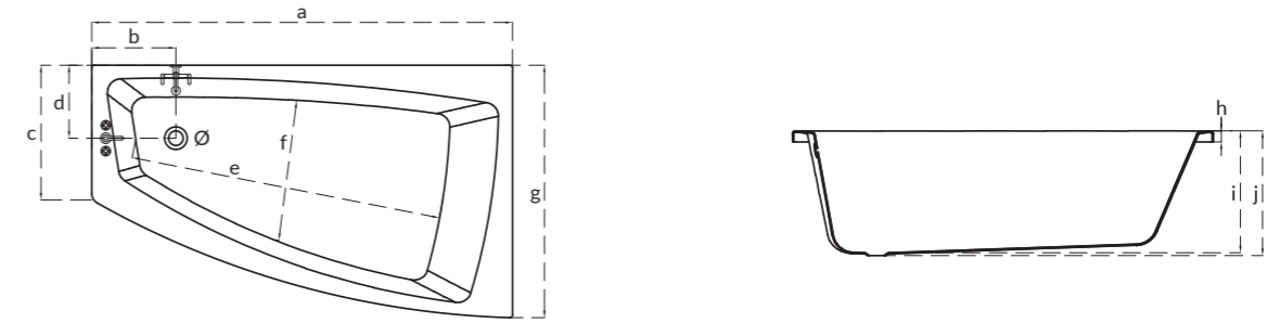
Асиметрична ванна LORENA, права, ліва LORENA asymmetric bathtub, right, left
