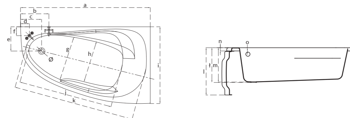
Асиметрична ванна JOANNA NEW, права, ліва JOANNA NEW asymmetric bathtub, right, left
