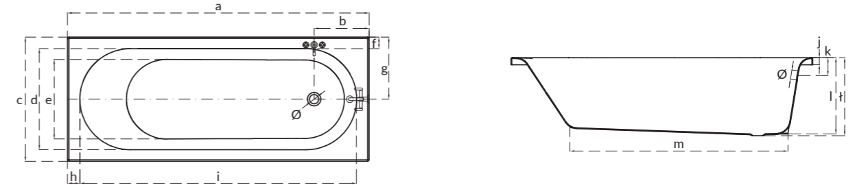
Прямокутна ванна OCTAVIA OCTAVIA rectangular bathtub
