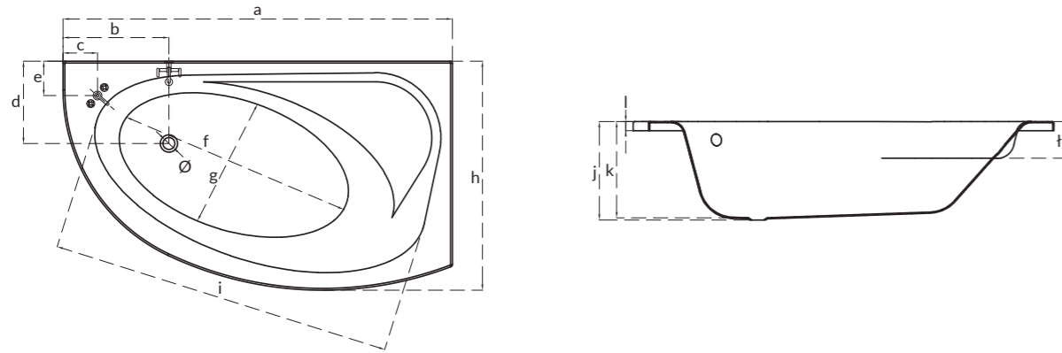
Асиметрична ванна MEZA, права, ліва MEZA asymmetric bathtub, right, left
