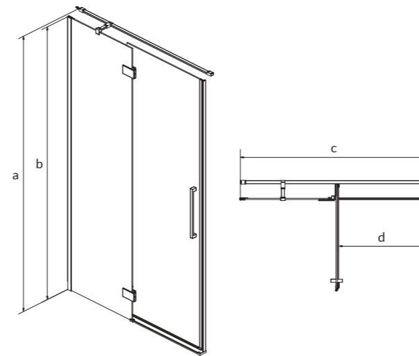
Душові двері розпашні CREA, лівосторонні CREA shower enclosure door with hinges, left
