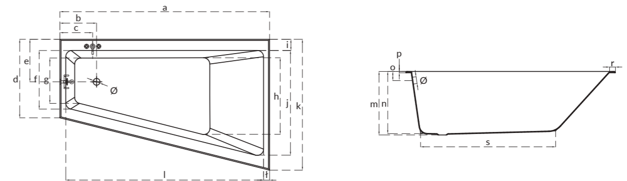
Асиметрична ванна CREA, права, ліва CREA asymmetric bathtub, right, left
