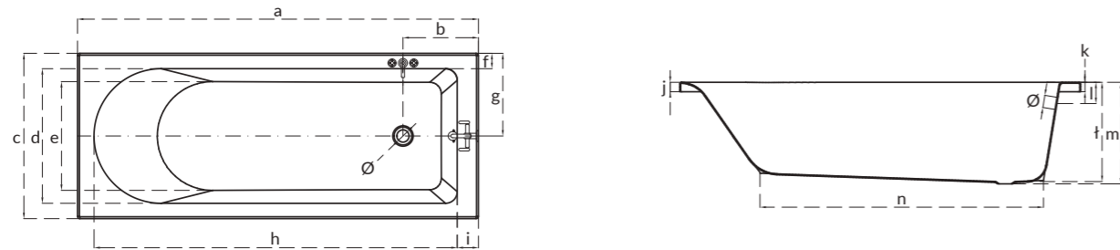
Прямокутна ванна FLAVIA FLAVIA rectangular bathtub
