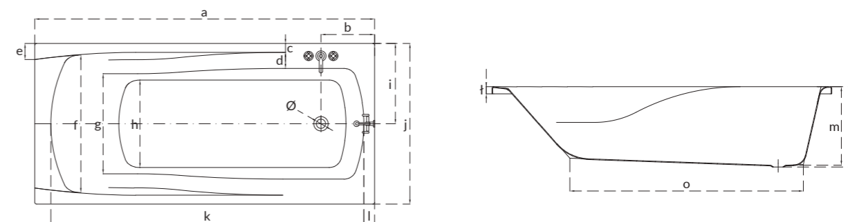
Прямокутна ванна ZEN ZEN rectangular bathtub
