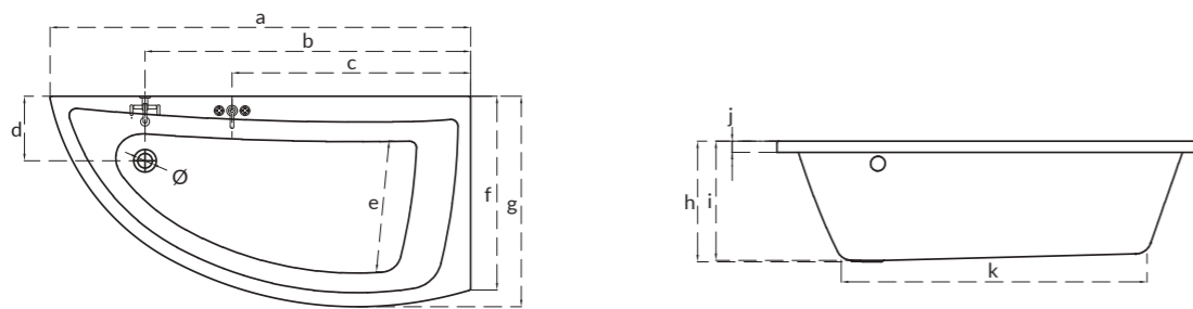
Асиметрична ванна NANO, права, ліва NANO asymmetric bathtub, right, left
