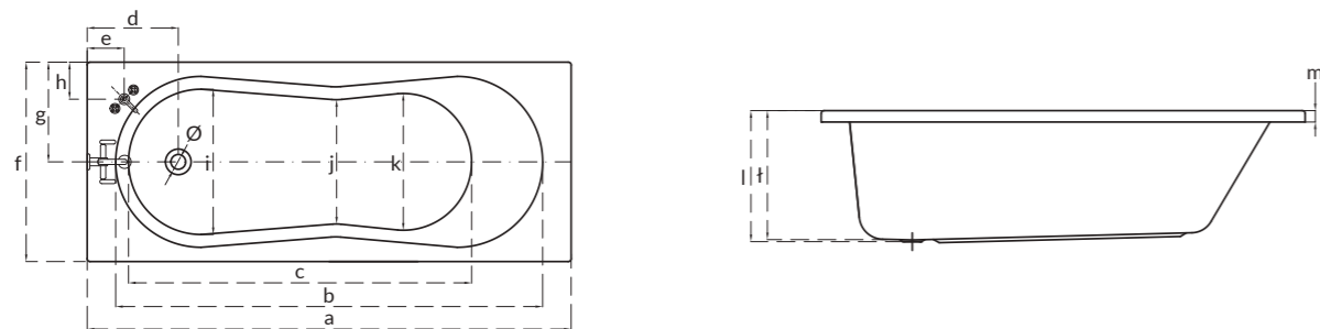
Прямокутна ванна NIKE NIKE rectangular bathtub
