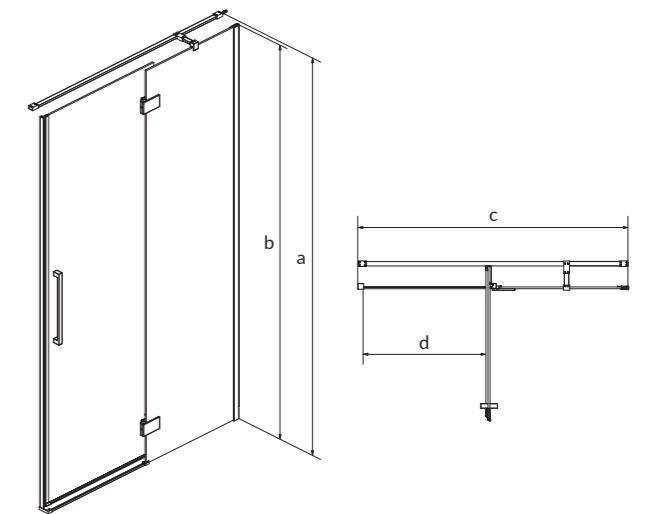
Душові двері розпашні CREA, правосторонні CREA shower enclosure door with hinges, right
