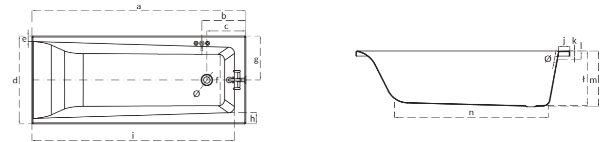
Прямокутна ванна LORENA LORENA rectangular bathtub
