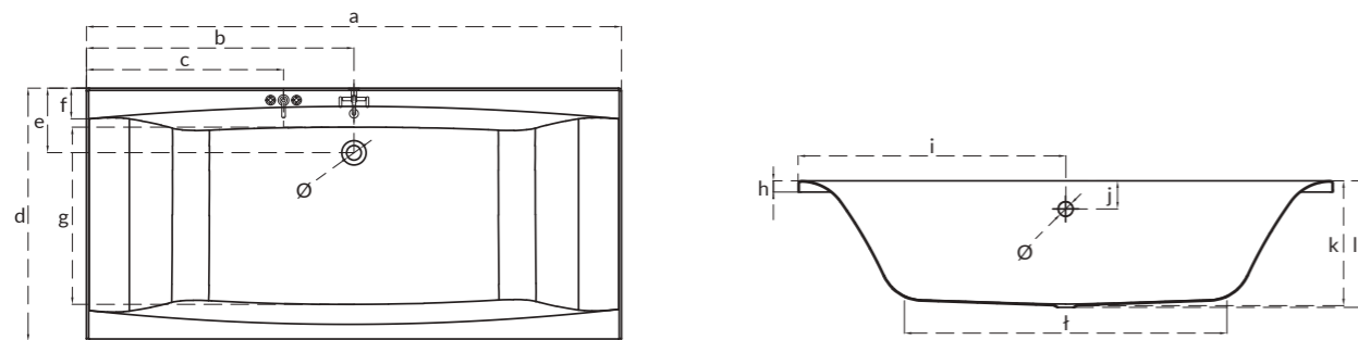
Прямокутна ванна VIRGO VIRGO rectangular bathtub
