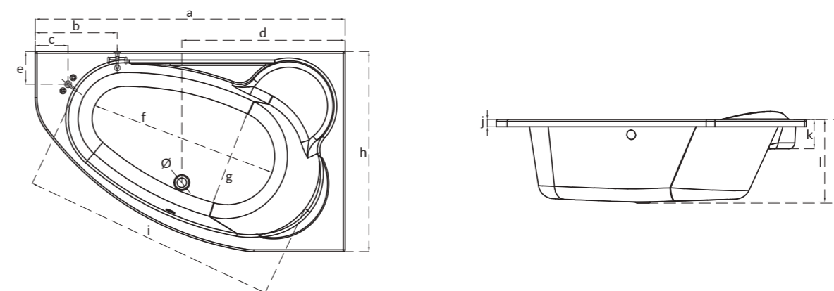
Асиметрична ванна KALIOPE, права, ліва KALIOPE asymmetric bathtub, right, left
