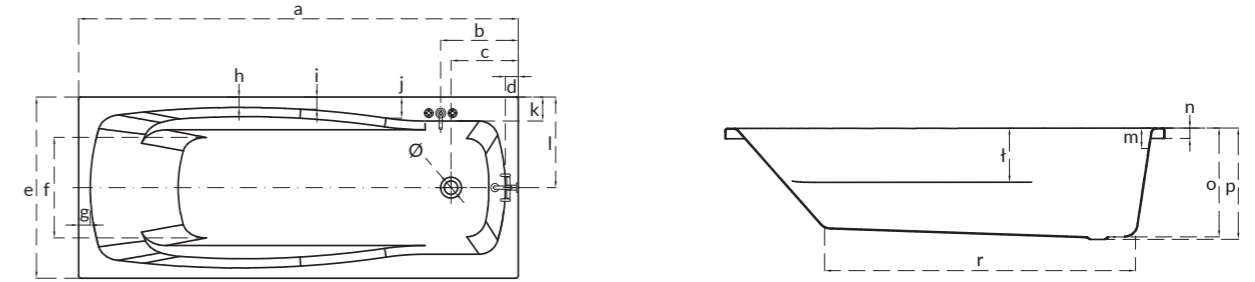
Прямокутна ванна LANA LANA rectangular bathtub
