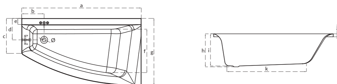
Асиметрична ванна VIRGO MAX, права, ліва VIRGO MAX asymmetric bathtub, right, left
