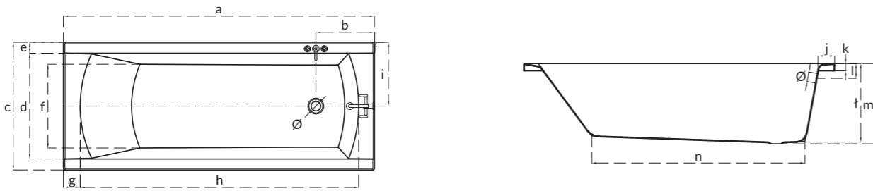
Прямокутна ванна KORAT KORAT rectangular bathtub
