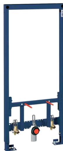
Инсталляция Rapid SL Grohe 49007
