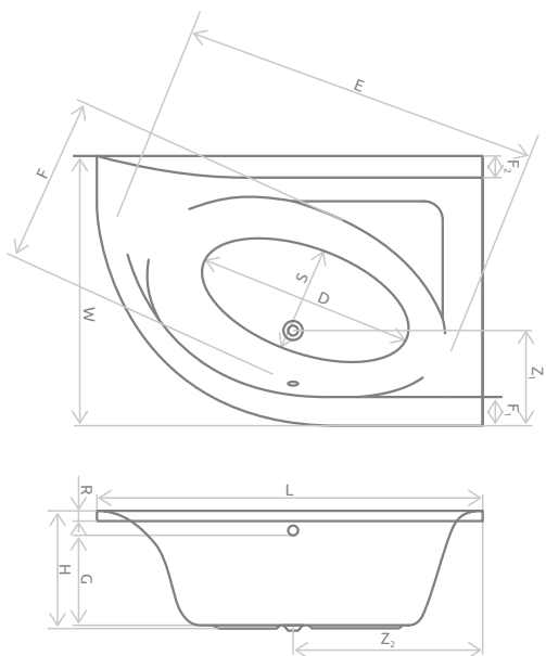
Розміри ванни, згідно схеми (мм)
