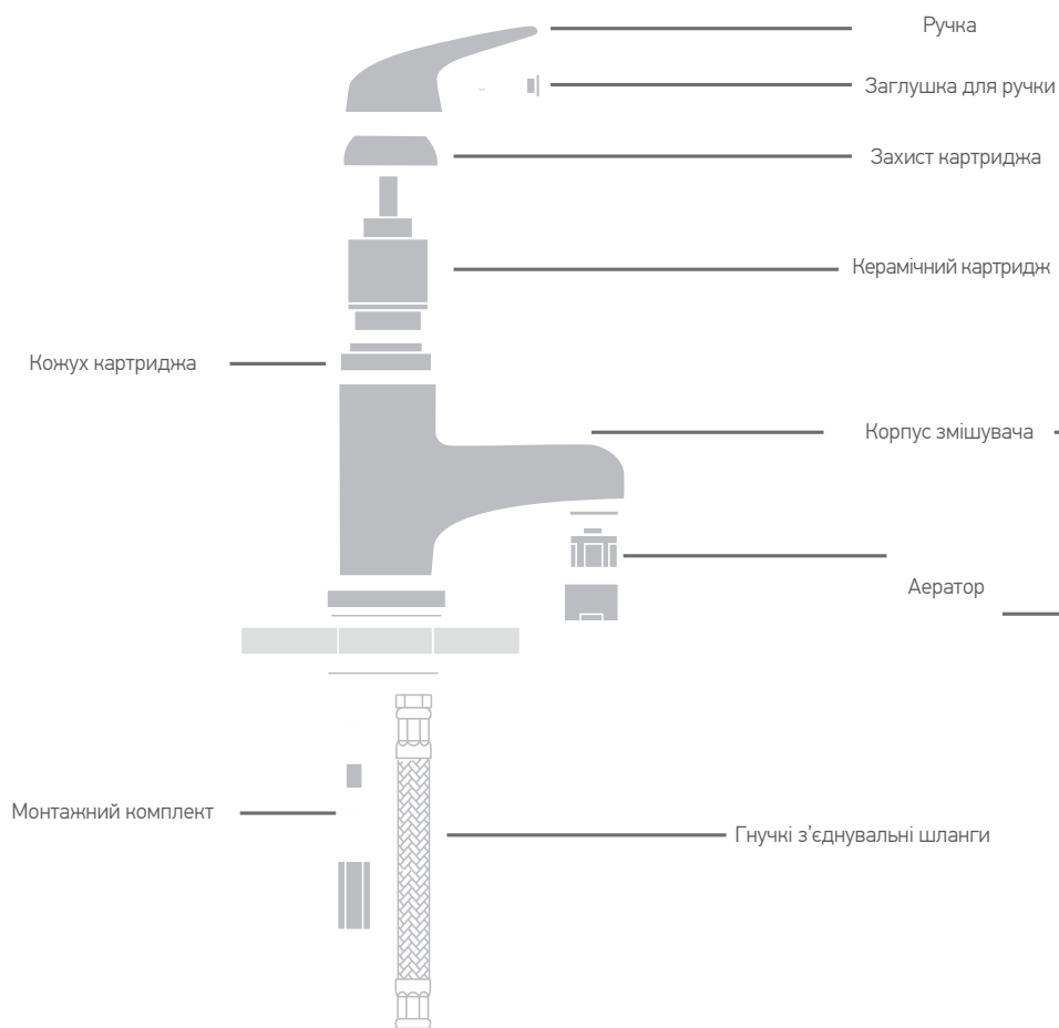
ЗМІШУВАЧ ДЛЯ УМИВАЛЬНИКА
