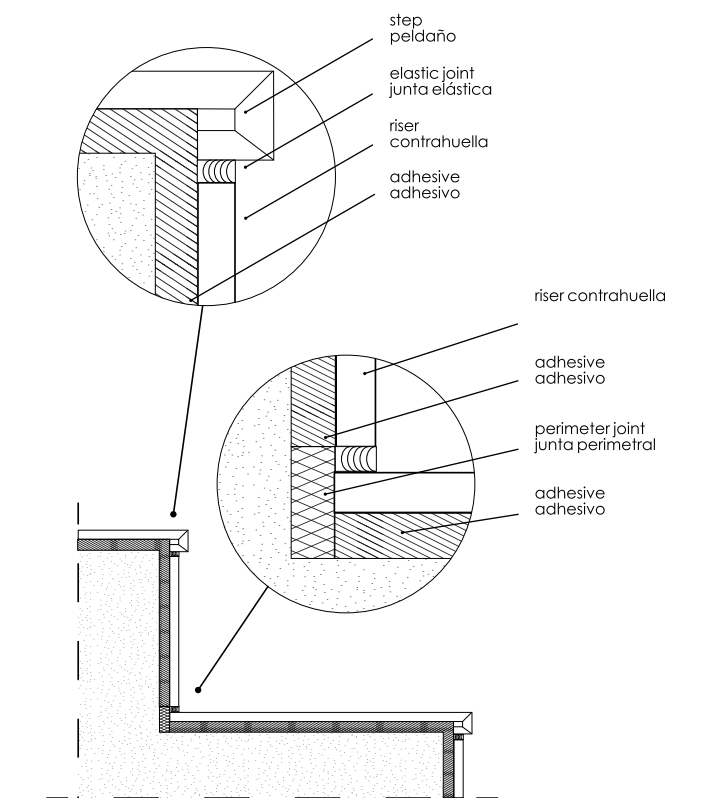
DETAIL OF STEPS ON A STAIRCASE | DETALLE DE PELDAÑOS EN ESCALERA (UNE 138002:2017)
