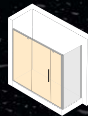
Раздвижная дверь с неподвижным сегментом и дополнительным элементом
