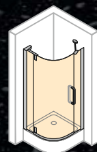
1/4 круга, односекционная распашная дверь с неподвижными сегментами
