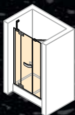
Распашная дверь с неподвижным сегментом и дополнительным элементом для ниши
