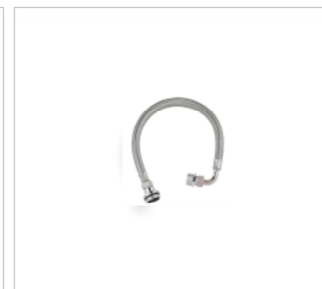
12 124 000 Grohtherm XL Подвод смешанной воды, гибкий присоединительный шланг 3/4" x 3/4", угол 90°, для подключения к водопроводу
