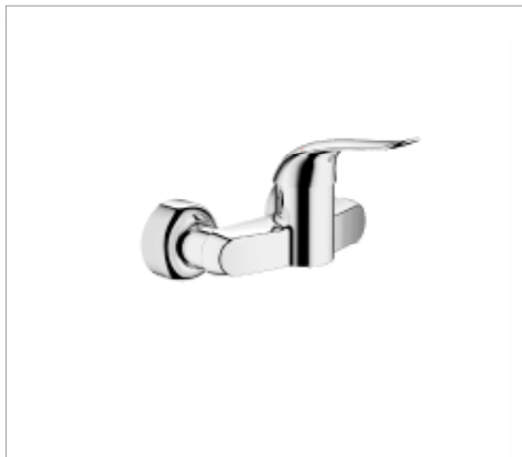
32 782 000 Euroeco Special Смеситель однорычажный для душа, DN 15, настенный монтаж, отвод для душа снизу 1/2", встроенный обратный клапан, регулировка расхода воды, металлический рычаг 120 мм, ограничитель температуры
