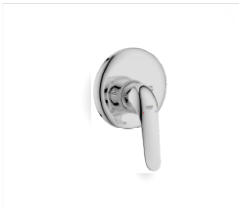
32 784 000 Euroeco Special Смеситель однорычажный для душа, DN 15, комплект верхней монтажной части для 35 501 000, металлический рычаг 120 мм, металлическая розетка, ограничитель температуры
