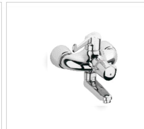
34 021 000 Grohtherm Ergomix Термостат для раковины, DN 15, с локтевым управлением, металлический рычаг 250 мм, рукоятка выбора температуры с предварительно устанавливаемым стопором безопасности, термическая дезинфекция, вынос 195 мм
