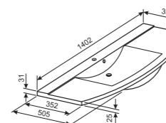
UM 140.118 Umivalnik Umivaonik Basin Waschbecken 152,45 PT *
