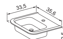
UM 35.183 Umivalnik Umivaonik Basin Waschbecken 92,13 PT *
