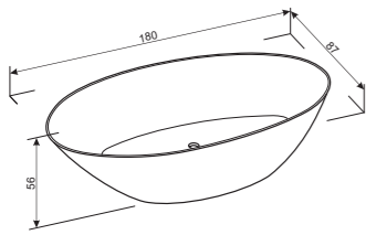
KK 156.04 L, D Kopalna kad luna Kada za kupanje luna Bathtub luna Badewanne luna 560,96 PT *
