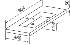
UM 80.95 Umivalnik Umivaonik Basin Washbecken 123,31 PT *
