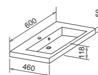
UM 60.95 Umivalnik Umivaonik Basin Waschbecken 113,78 PT *
