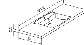
UM 121.110 Umivalnik Umivaonik Basin Waschbecken 146,60 PT *
