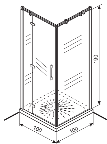
KTK 100.37 Kaljeno prozorno steklo z Antiplaque premazom Kaljeno prozorno staklo s premazom Antiplaque Tempered transparent glass with Antiplaque coating gehärtetes Klarglas mit Antiplaque Beschichtung 865,37 PT *
