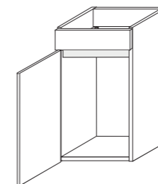
F 40.02 L,D Element pod umivalnikom Element ispod umivaonika Vanity cabinet Waschbeckenunterschrank • 40/50/21,6 61,86 PT *
