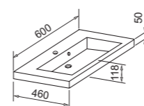
UM 60.95 Umivalnik Umivaonik Basin Waschbecken 113,78 PT *
