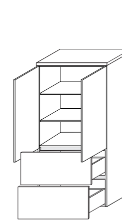
BKG 60.38 Visoka omara s pokrivno ploščo Visoki ormar s pokrovnom pločom Tall cabinet with functional top Hochschrank mit Deckplatte • 60,2/126,6/36 217,43 PT *
