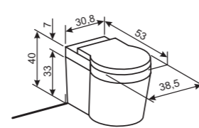
WC 39.27 WC školjka Julija WC školjka Julija Toilet bowl Julija Toilettenschüssel Julija • 38,5/43,5/53 531,76 PT *
