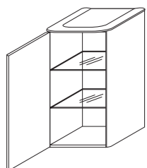
BKG 35.21 L,D Spodnji element z odlagalno polico iz kompozitnega materiala L,D Donji element s policom za odlaganje, od kompozitnoga materijala L,D Base cabinet with functional top made of composite material L,R Unterschrank mit Ablage aus Kompositmaterial L,R • 35,6/75/33,5 209,05 PT *
