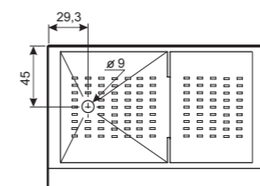
KTK 160.75 Tuš kabina Kuba Kaljeno prozorno steklo z Antiplaque premazom Kaljeno prozorno staklo s premazom Antiplaque Tempered transparent glass with Antiplaque coating gehärtetes Klarglas mit Antiplaque Beschichtung 1.300,78 PT *
