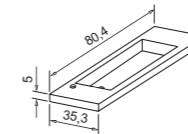
UM 80.120 Umivalnik Umivaonik Basin Waschbecken 80,4/5/35,3 131,68 PT *
