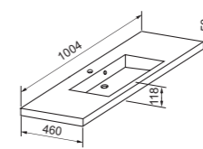
UM 100.95 Umivalnik Umivaonik Basin Waschbecken 139,76 PT *
