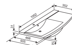
UM 105.118 L Umivalnik, levi Umivaonik, lijevi Basin, left Waschbecken, links 128,98 PT *
