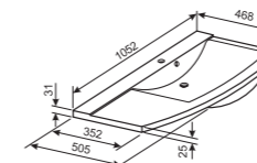
UM 105.118 D Umivalnik, desni Umivaonik, desni Basin, right Waschbecken, rechst 128,98 PT *
