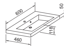
UM 60.95 Umivalnik Umivaonik Basin Washbecken 113,78 PT *
