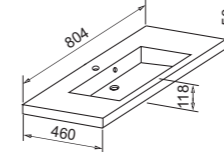
UM 80.95 Umivalnik Umivaonik Basin Waschbecken 123,31 PT *
