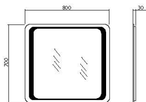
Омега 80 / Omega 80
