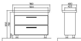
Паола 100 / Paola 100
