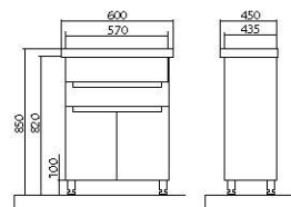
Омега 60 / Omega 60
