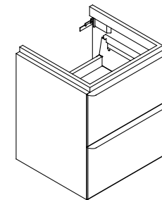
4.1010.2 X. 435 mm Y. 520 mm Z. 410 mm
